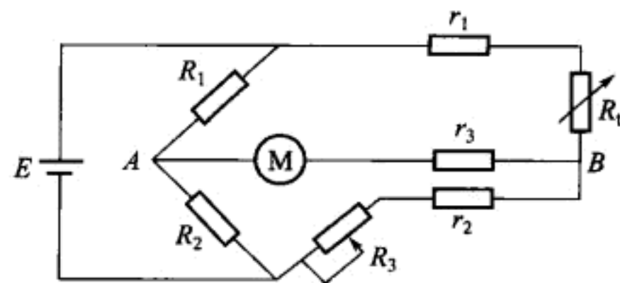
图 2-31 热电阻测温电桥的三线连接
