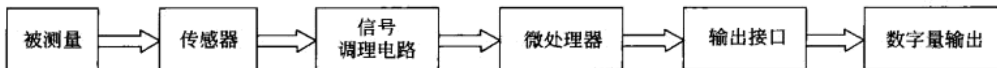
图 2-38 智能传感器结构框图
