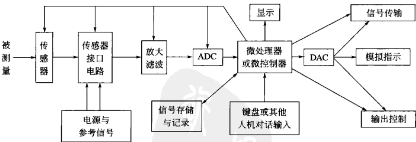
图 1-2 测控系统的一般结构
