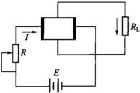
图 2-34 霍尔元件的基本电路
