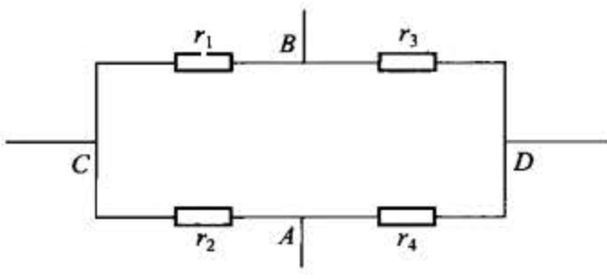
图 2-36 霍尔元件的等效电路
