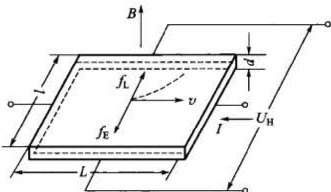
图 2-32 霍尔效应原理
