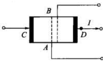
图 2-35 不等位电势示意图
