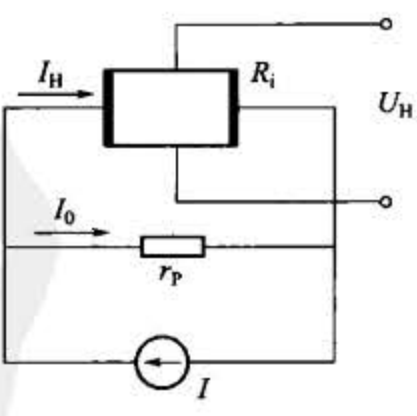
图 2-37 温度补偿线路
